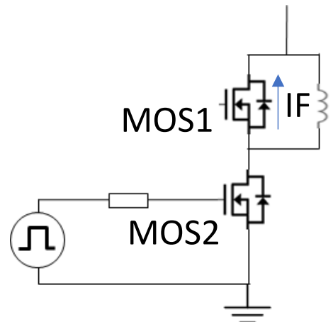
Fig.6 开关电路示例 当电流流过 MOS2，然后关闭时，中频电流流过 MOS1。当 MOS2 再次开启时，该电流流过 MOS2 电流流过 MOS2 时，MOS1 的体二极管的电压会升高。MOS1 的体二极管电压上升，显示出反向恢复操作，电流波形如图 5 所示。电流波形如图 5 所示。
